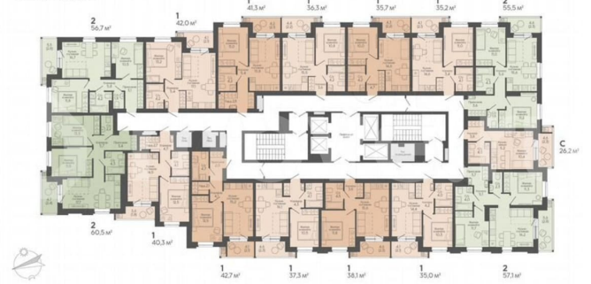
Типовые этажи 2-12
